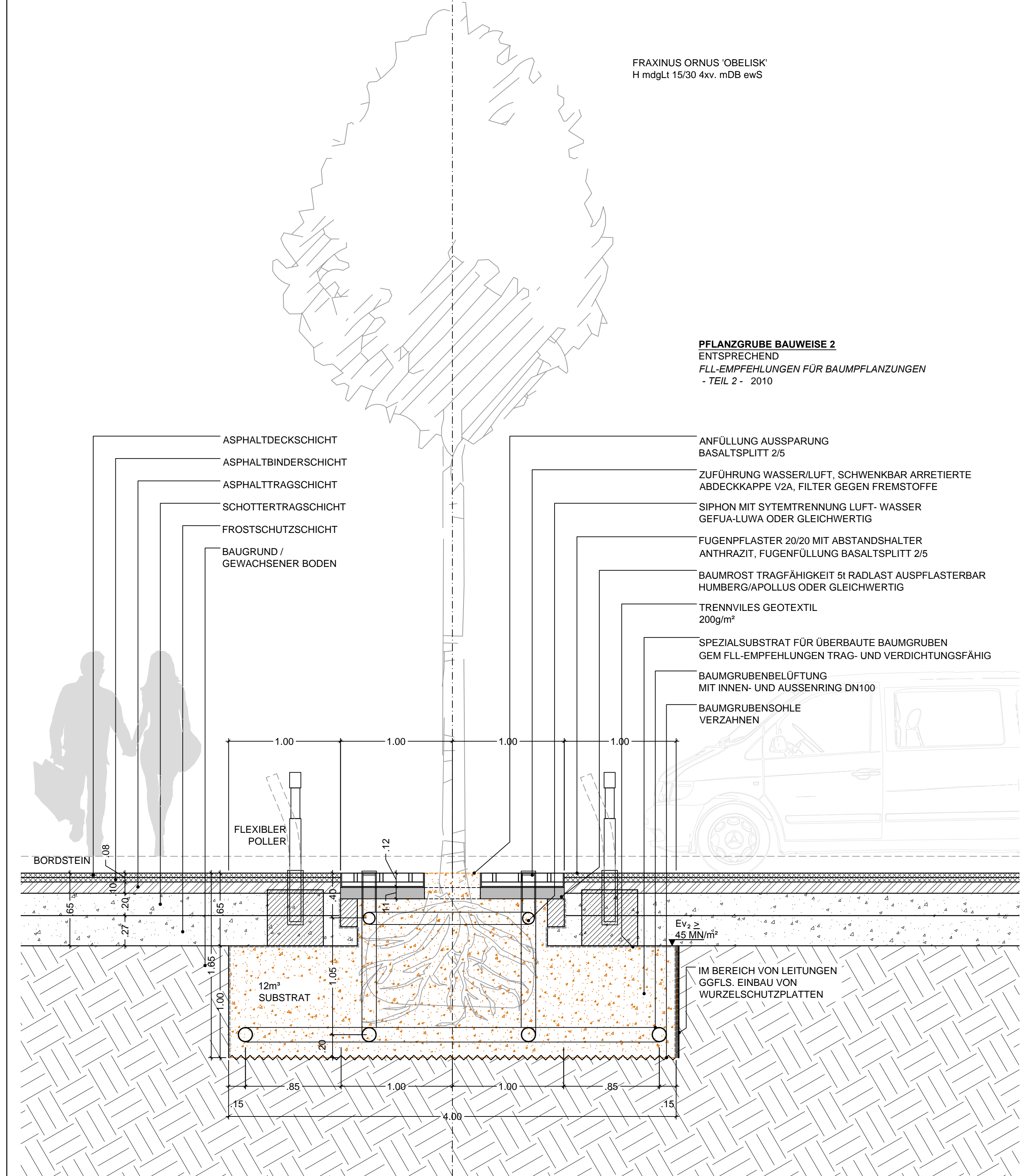
DETAIL BAUMSTANDORT M 1:25
